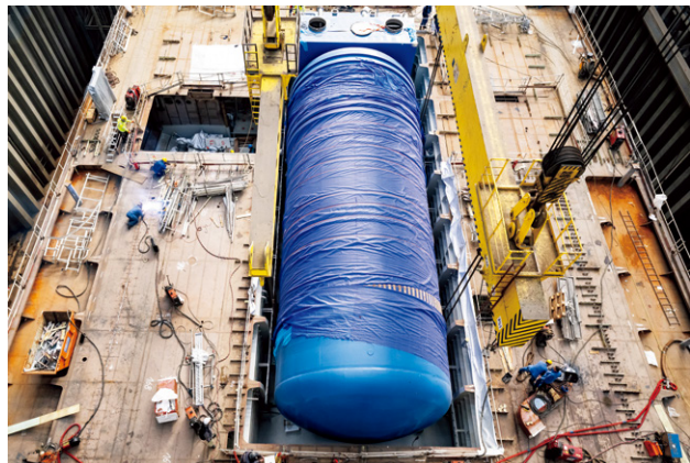
船体に設置されるLNGタンク。重油・軽油・ナチュラルガスの計3種の燃料を使用できるトリフューエルエンジンを搭載
